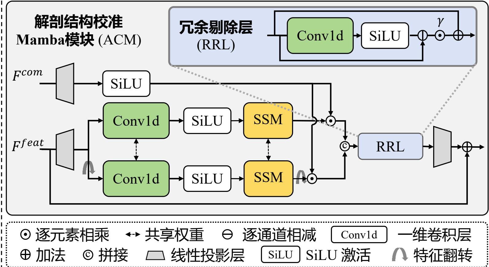
(b) ACM 模块示意图
