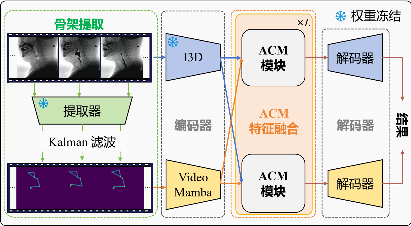
(a) AC-Mamba框架示意图
